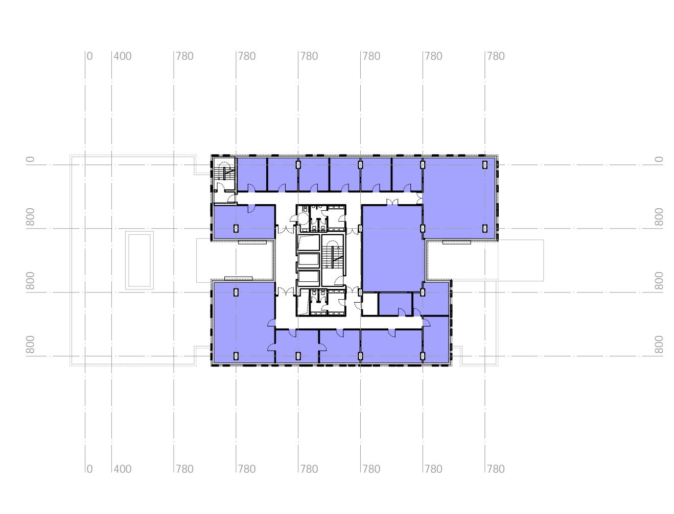
OSNOVA +18. SPRATA
