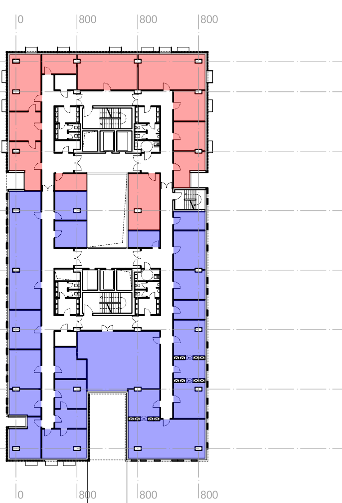
OSNOVA +4. SPRATA
