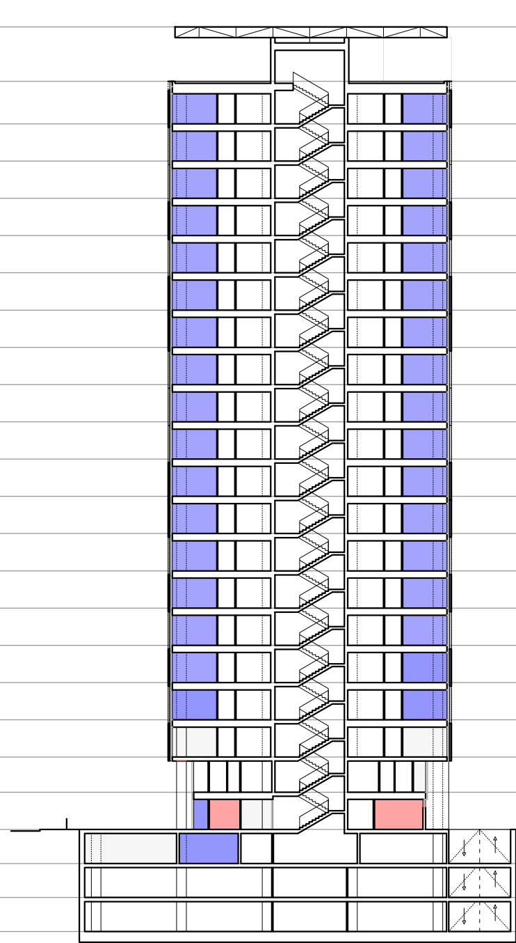
PRESJEK C-C
