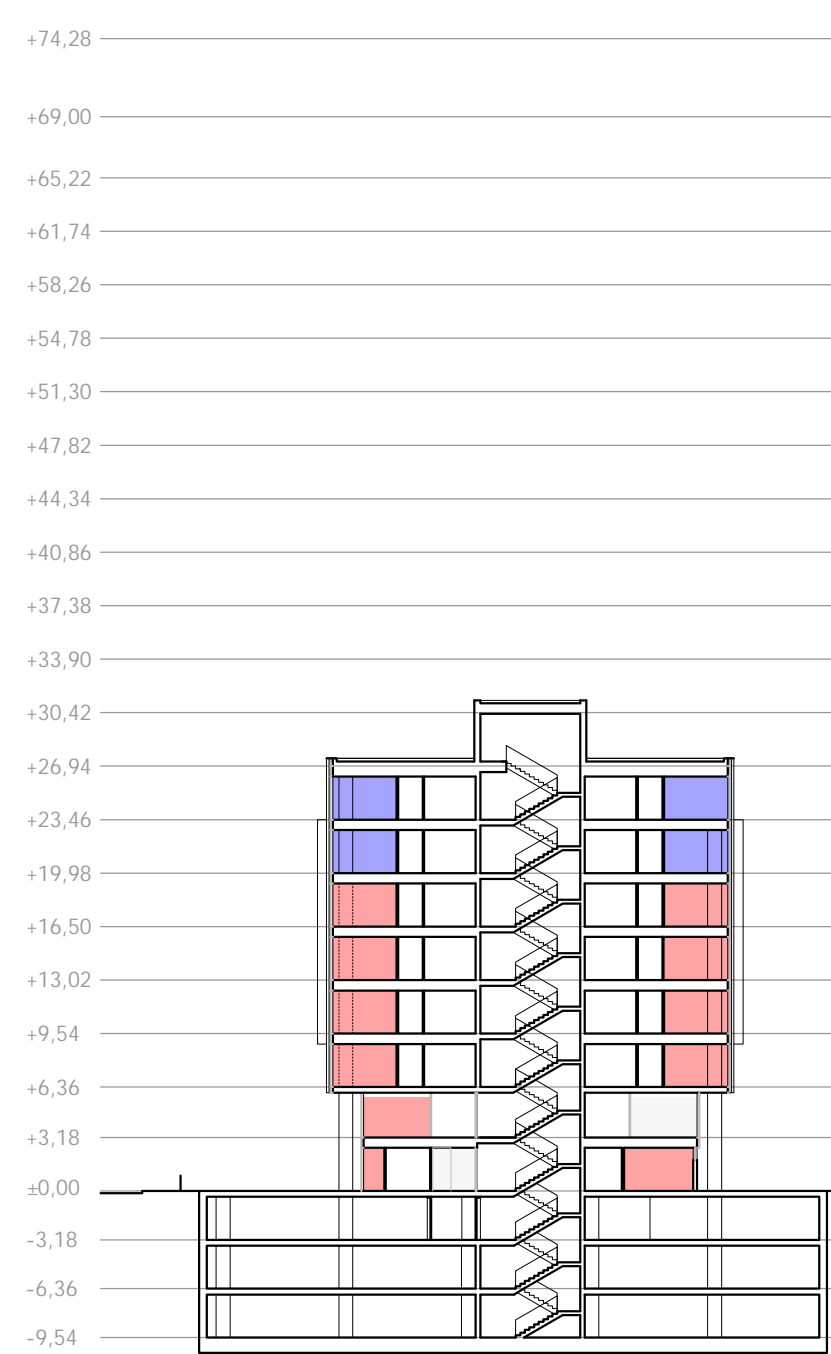
PRESJEK A-A
