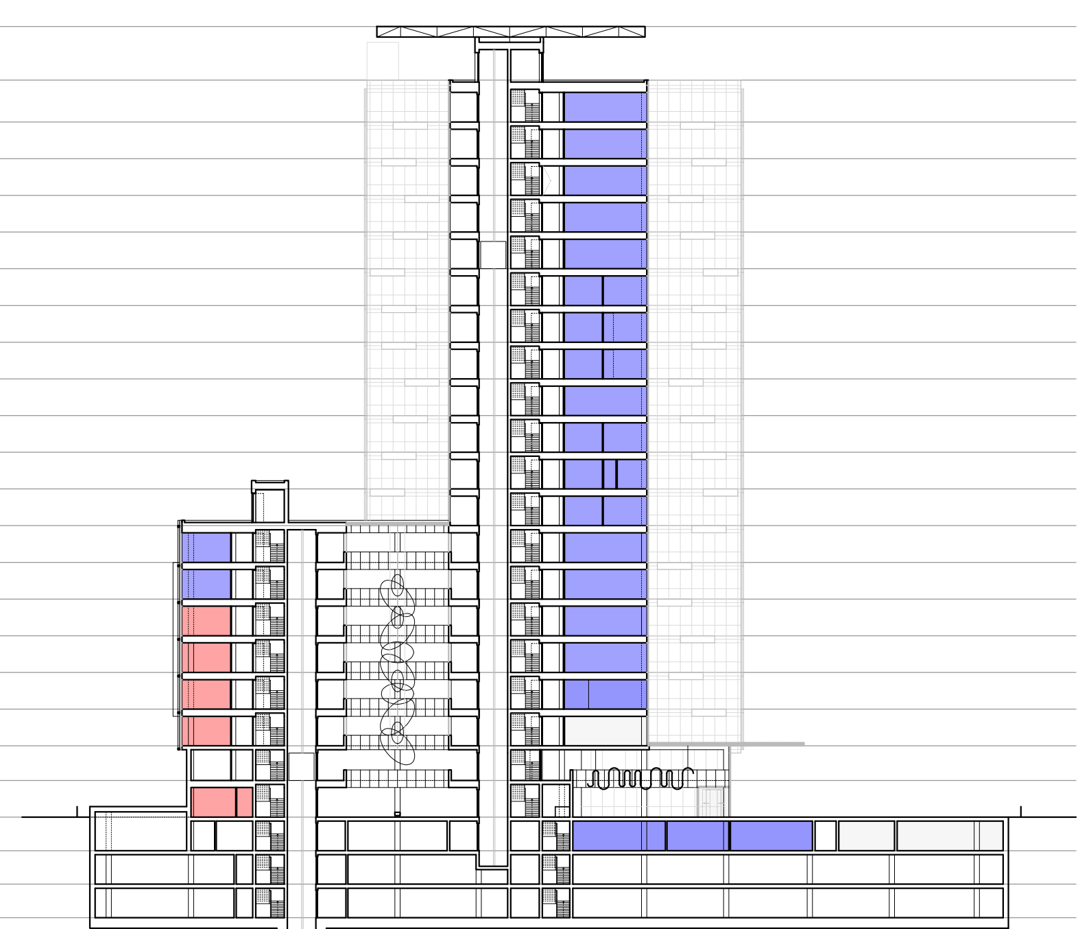
PRESJEK E-E
