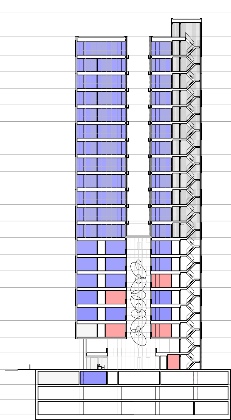
PRESJEK B-B
